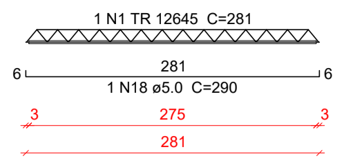
VT209a (3 unidades) (L209) ESC 1:50
