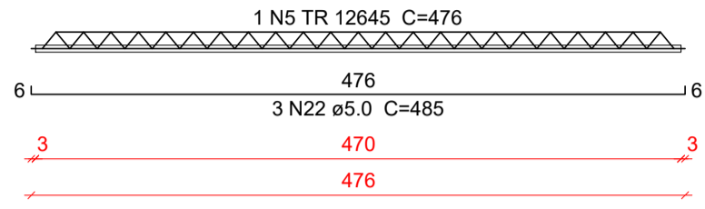
VT216a (9 unidades) (L216) ESC 1:50
