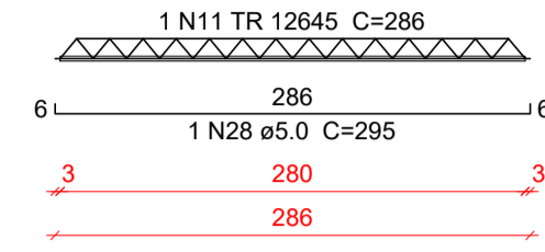
VT213a (33 unidades) (L213) ESC 1:50
