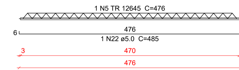
VT213a (33 unidades) (L213) ESC 1:50
