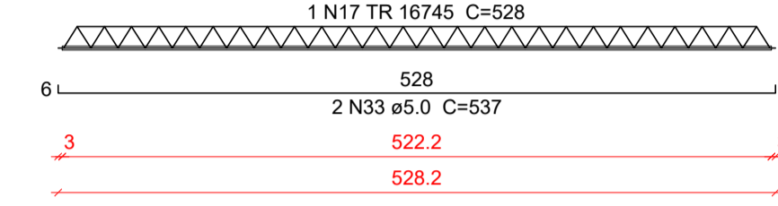
VT220a (7 unidades) (L220) ESC 1:50
