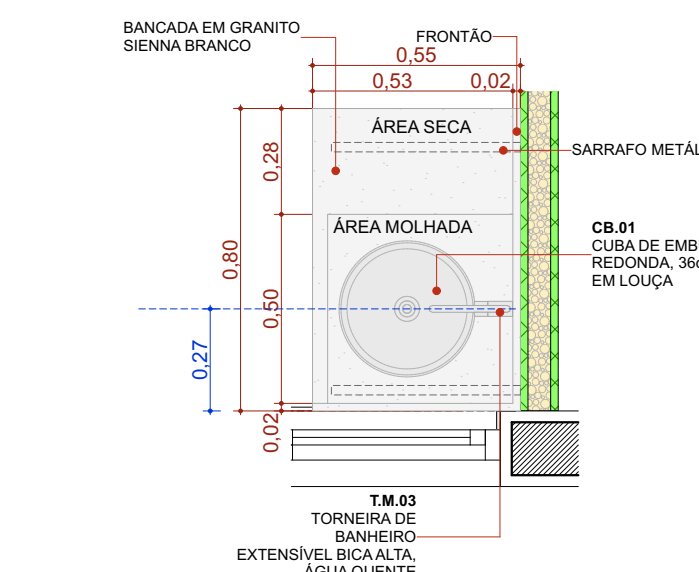
BPC.80d Escala:1:20
