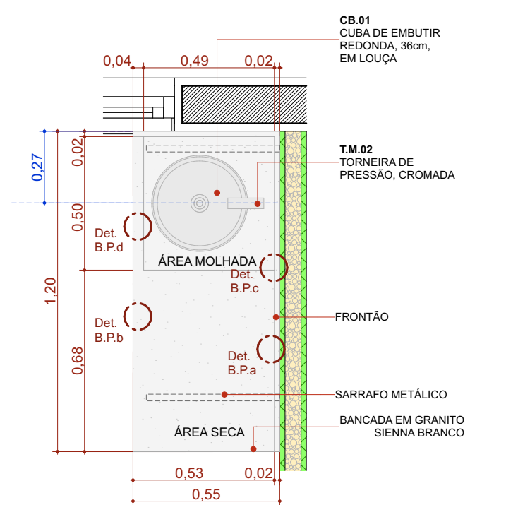
BPC.120e Escala:1:20
