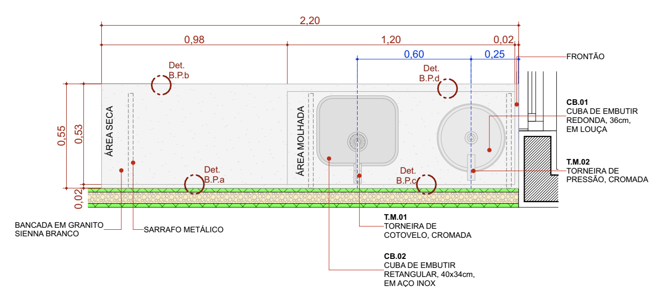
BPC.220e Escala:1:20
