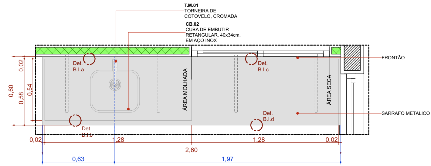
BIC.260d Escala:1:20
