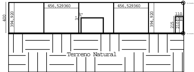
Corte A-A
