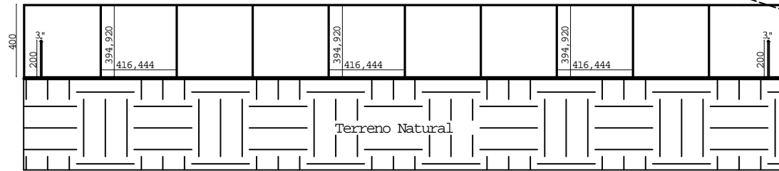
Corte A-A
